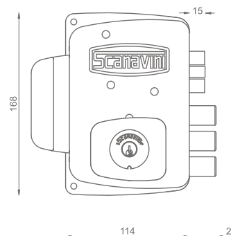
Dimensiones (mm)
